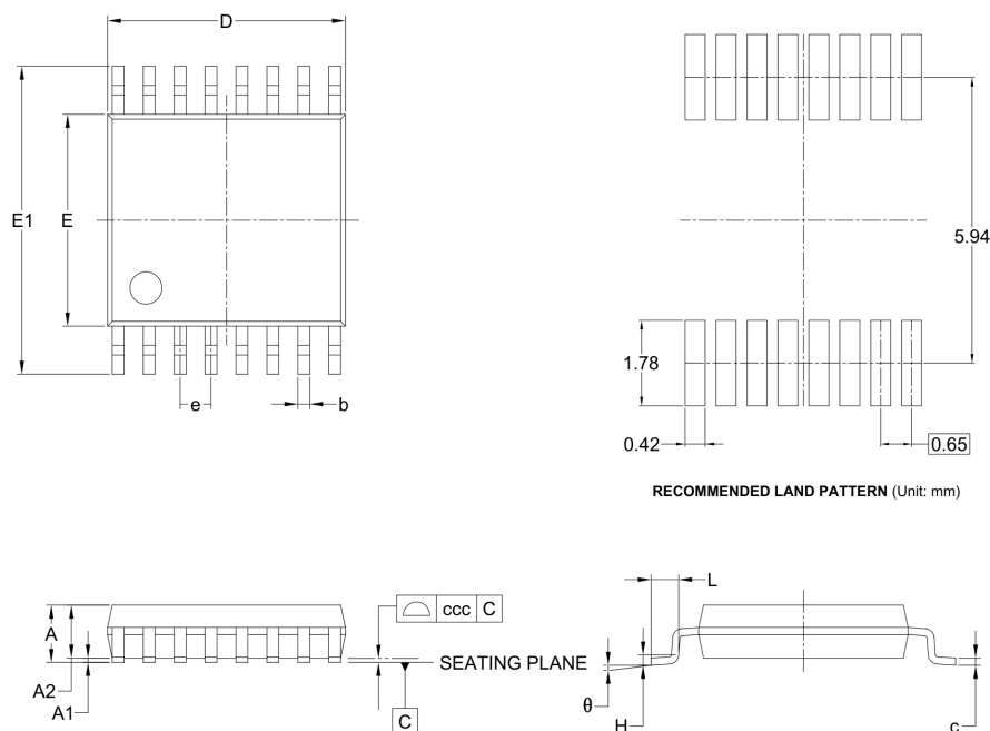
TSSOP-16
